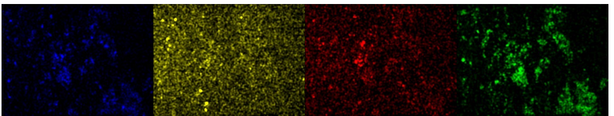
Hărți compoziționale ale radiației Röntgen secundare pentru Nb, Th, Y și Zr a câmpului din imaginea precedentă
