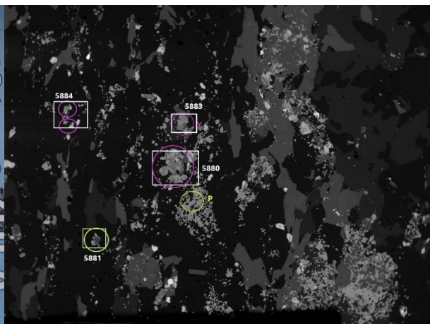
Imagine de electroni respinși a unui gnais microclinic cu metale rare
